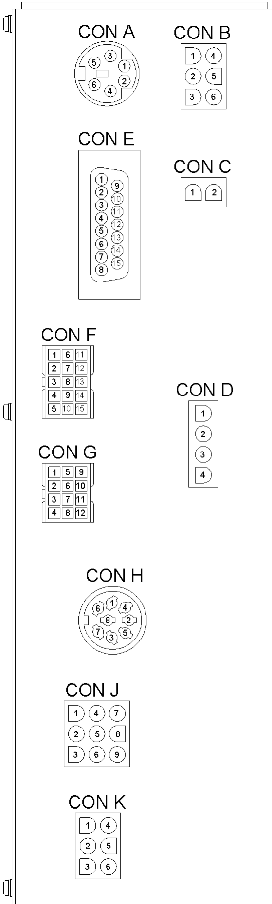
〔制御盤背面〕
