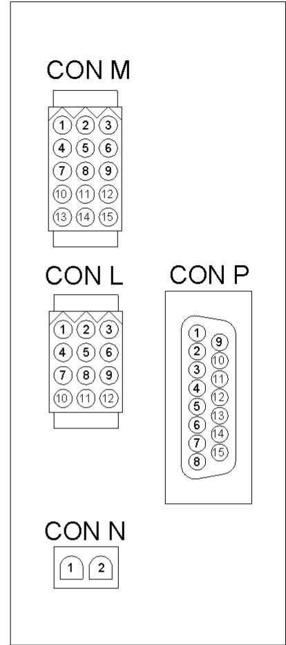
〔マシン背面〕
