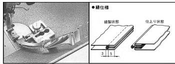
バイピングホルダー
