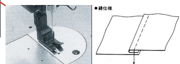
左段押え
