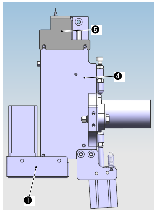
Dispositivo de la cuchilla móvil
