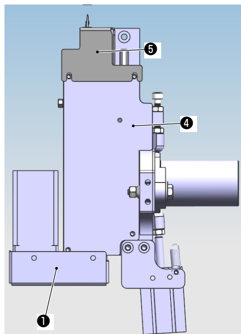
Dispositif du couteau mobile
