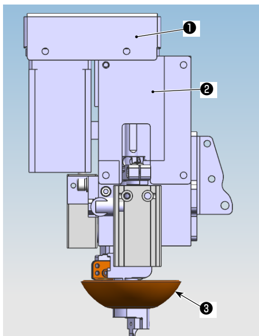
Dispositif du couteau fixe
