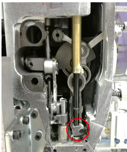
Vis de fixation pour le raccordement de la barre à aiguille
