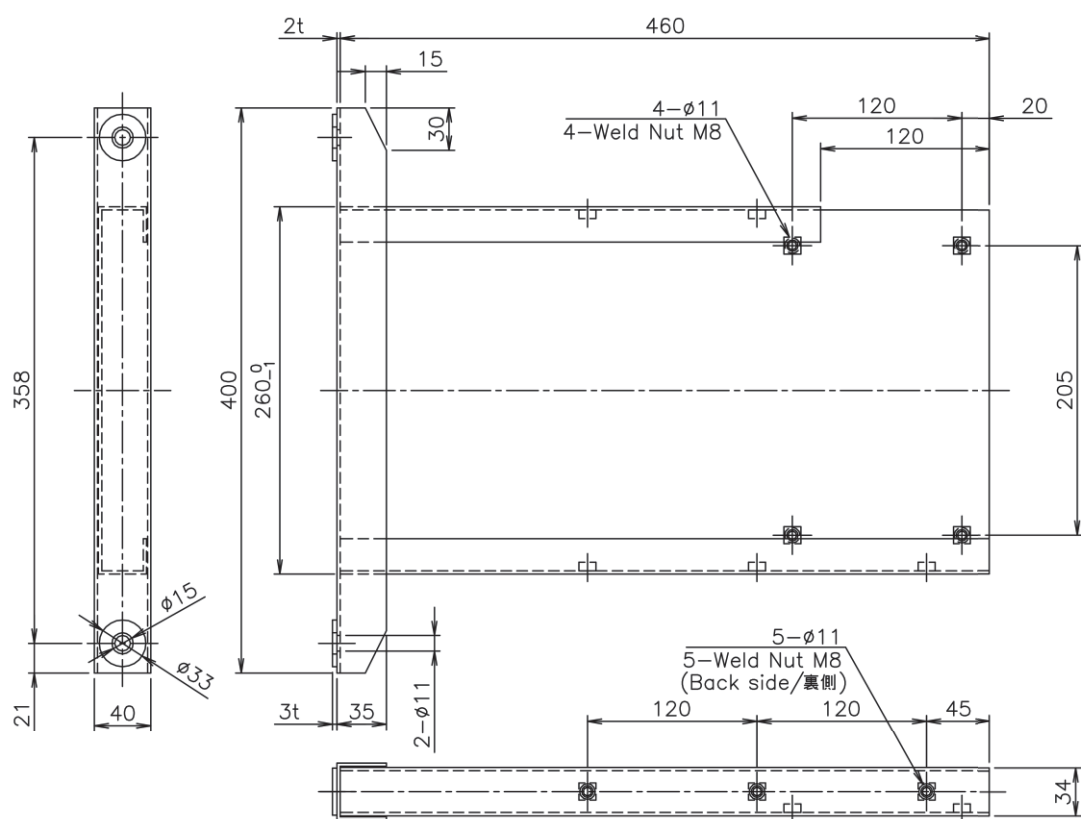
脚部品<2>・・・板厚 2 mm
