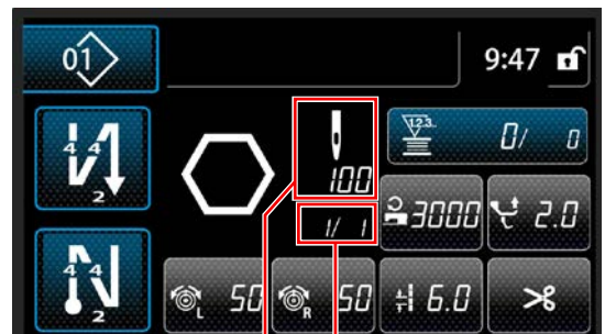
Çokgen şekilli dikiş deseni (Operatör modu)
