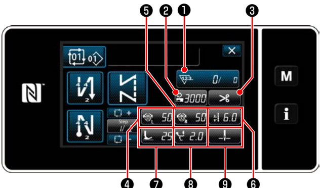
< 缝制画面（循环模式）>
