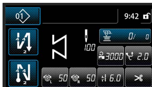
固定尺寸缝制图案（操作人员模式）
