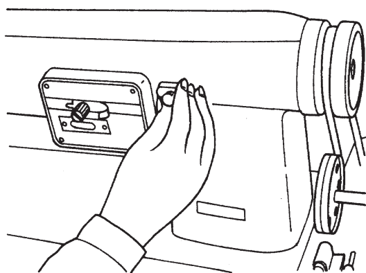
図 13 ③送りのつまみを上げる
