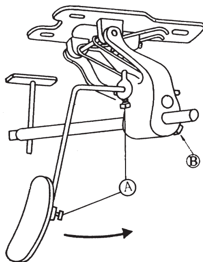
Fig. 32 Movimiento de palanca accionada por la rodilla
