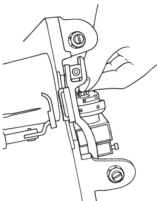
Fig. 24 Manera de sostener el fiador del portabobinas
