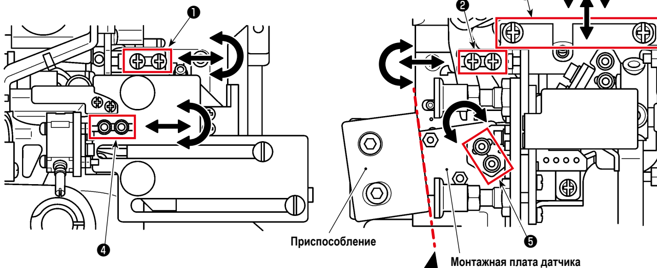
Рис. 1 Точки регулировки положения датчика
