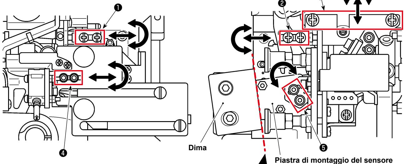
Fig. 1 Punti di regolazione della posizione del sensore
