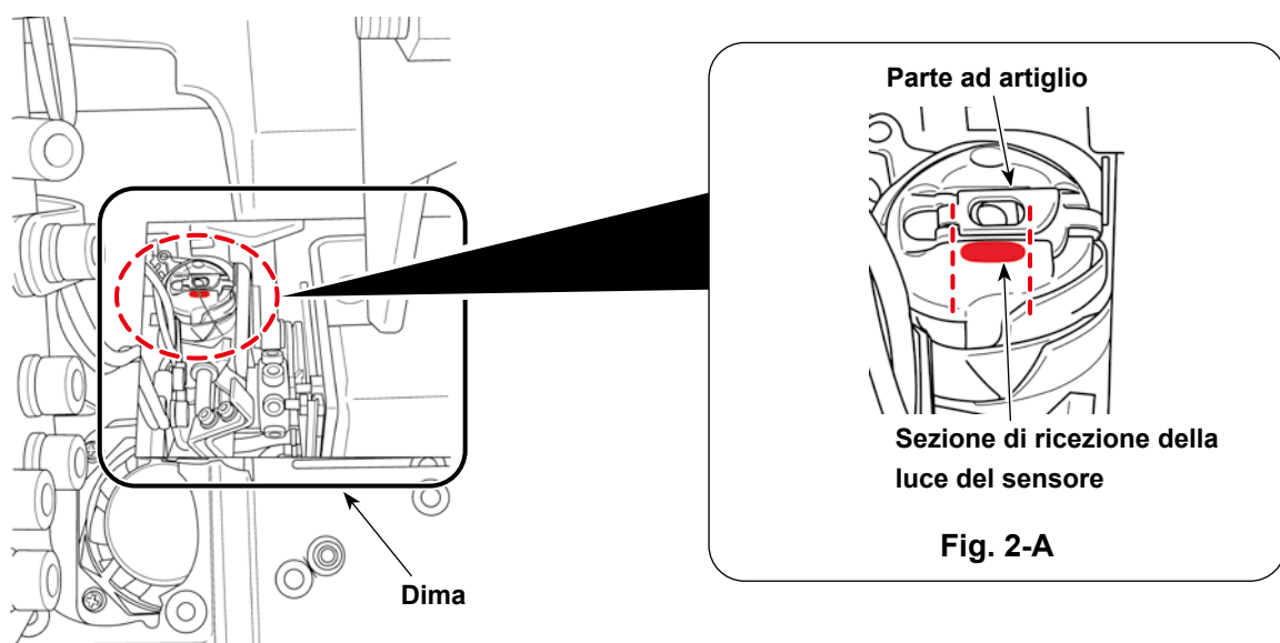
Fig. 2. Posizione di irradiazione della luce del sensore
