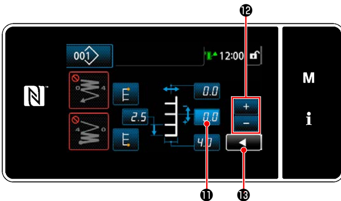
<Deuxième écran de couture>
