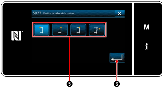
<Écran de sélection de la position de départ de la couture>
