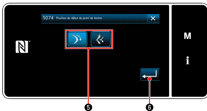
<Écran de sélection de la position de départ du point de feston>
