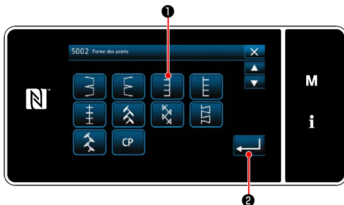
<Écran de sélection de la forme de couture>
