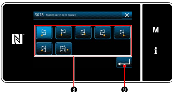
<Écran de sélection de la position de fin de couture>
