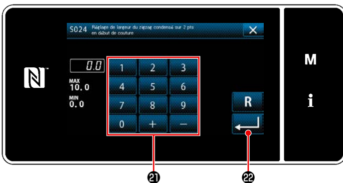
<Écran de réglage de la largeur de la couture condensée 2 points en début de couture>
