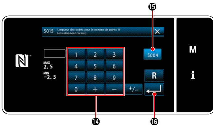
<Écran de saisie de la longueur des points (entraînement normal)>
