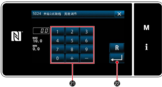
< 缝纫开始 2 点缩缝宽度调节画面 >
