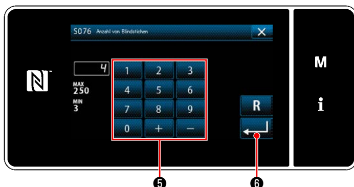
<Blindstichzahl-Eingabebildschirm>
