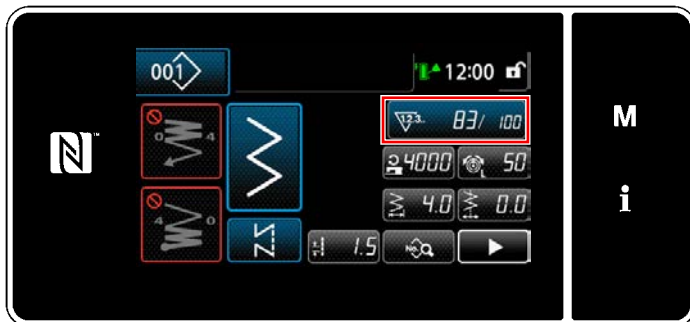
<Nähbetriebsbildschirm (Zähler)>
