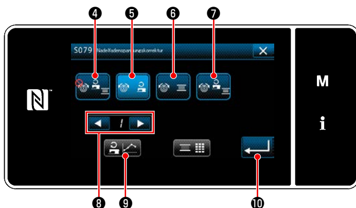
<S079 Nadelfadenspannungs-Korrekturbildschirm>
