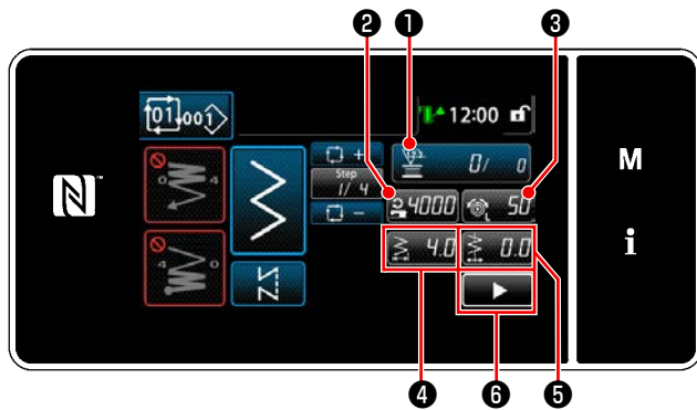
<Nähbetriebsbildschirm (Zyklusmodus)>
