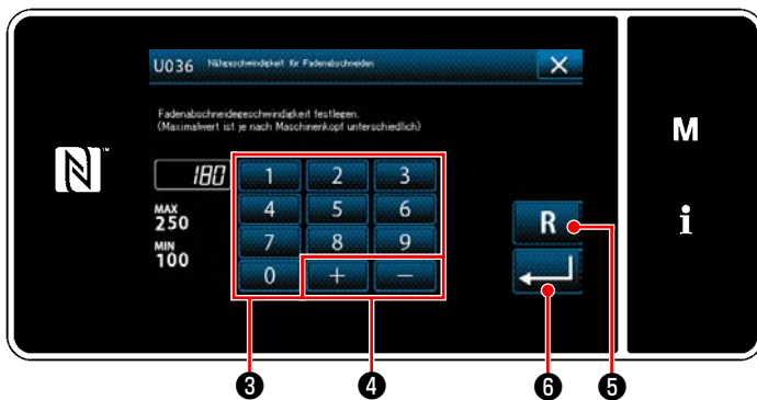
<Eingabebildschirm>
