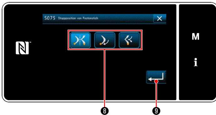
<Feststich-Stoppositions-Auswahlbildschirm>
