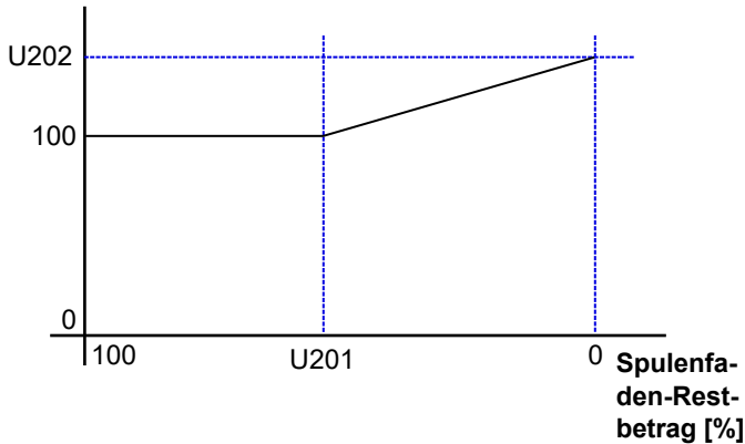
Spannungskorrekturbetrag [%]
