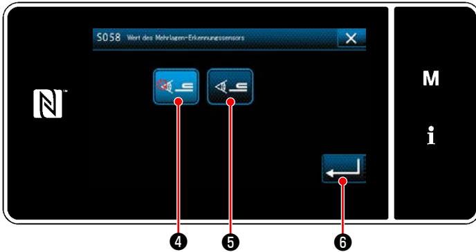
<Bildschirm für Mehrlagenabschnitt-Erkennungssensorwert>
