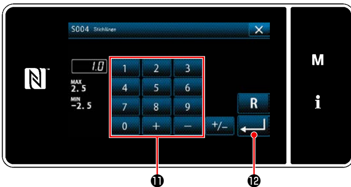
<Stichlängen-Eingabebildschirm>
