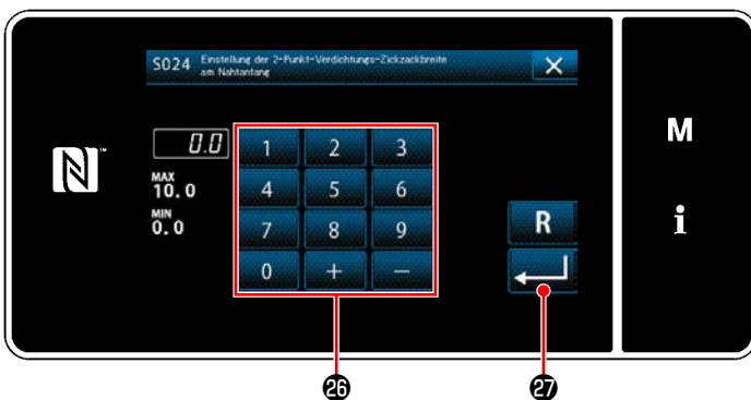
<Einstellbildschirm für 2-Punkt-Verdichtungsstichbreite am Nahtanfang>
