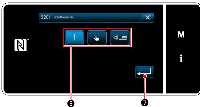
<Schrittschaltungsreferenz-Auswahlbildschirm>
