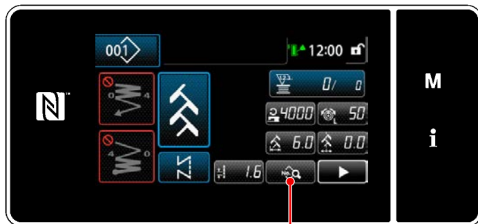
<Nähbetriebsbildschirm> ❸
