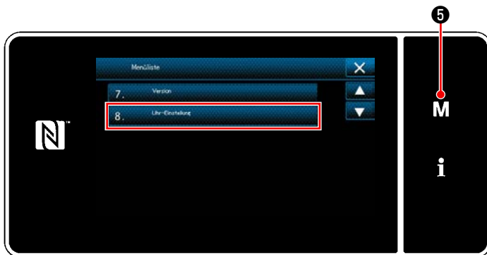
<Modusbildschirm>
