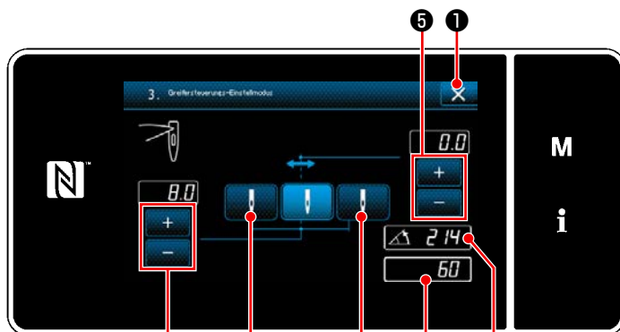
<Modusbildschirm>
