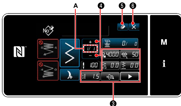
<Bildschirm zur Bearbeitung eines neuen Nähmusters> ③
