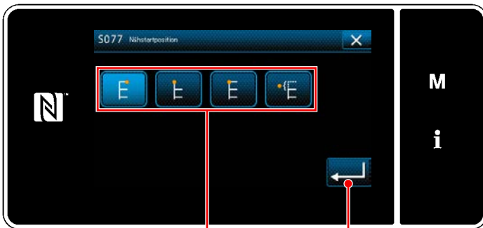
<Nähstartpositions-Auswahlbildschirm>
