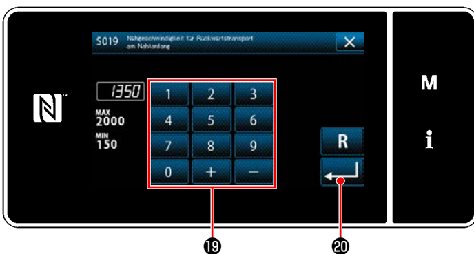
<Nähgeschwindigkeits-Eingabebildschirm für Rückwärtsnähen>
