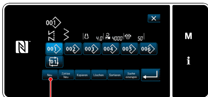
<Nähmuster-Listenscreen>
