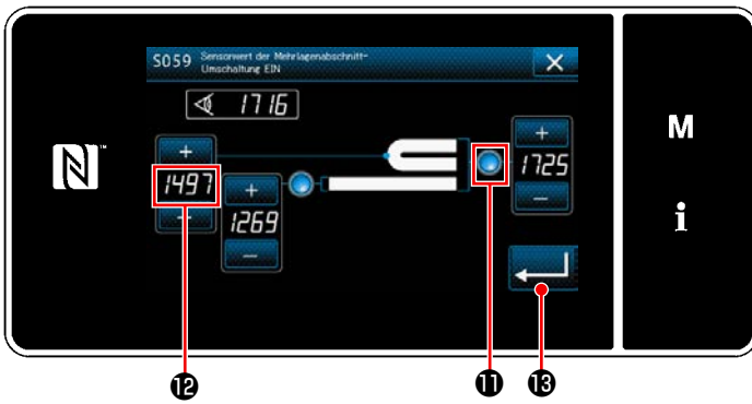
<Bildschirm zum Einlernen des Sensorwerts zum Einschalten der Mehrlagenabschnitt-Umschaltfunktion>
