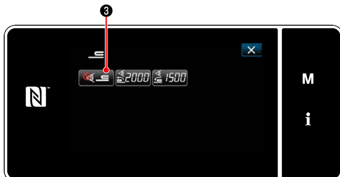
<Mehrlagenabschnitterkennung-Einstellbildschirm>
