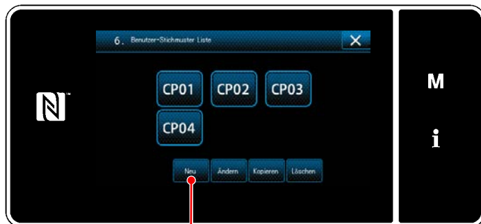
<Sondermuster-Listenbildschirm>
