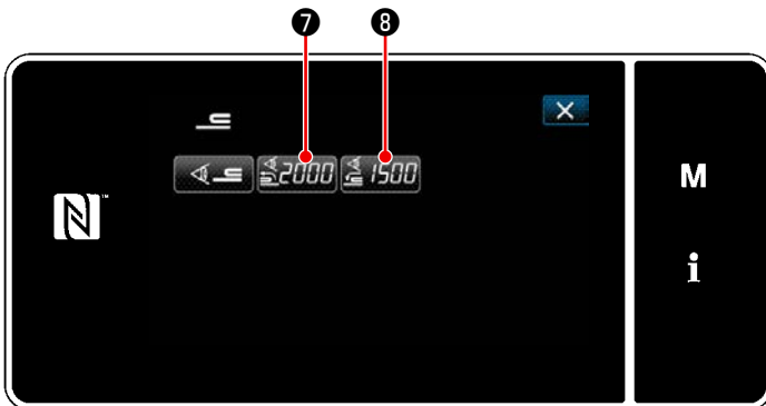
<Mehrlagenabschnitterkennungs-Einstellbildschirm>
