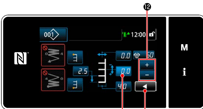
<Zweite Nähbetriebsbildschirm>
