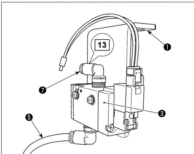
Valvola solenoide asm._AE (per il dispositivo di rilevamento della quantità rimanente del filo della bobina)
