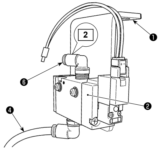
Valvola solenoide asm._SD (per il dispositivo di rilevamento dei salti di punto)
