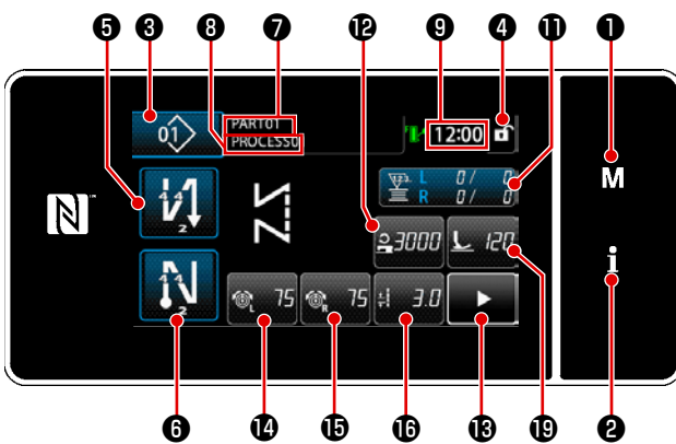
自由縫紉图案（操作人员模式）
