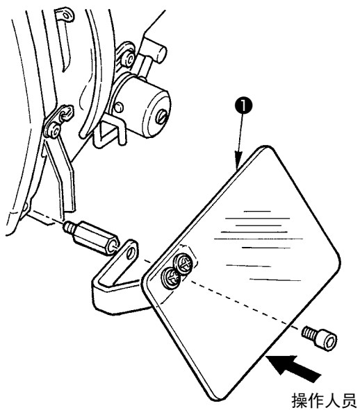
横向设置时
