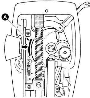
Position zur Prüfung der Ölmenge (Ölspritzer)
