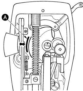
Posición para confirmar la cantidad de aceite (manchas de aceite)
