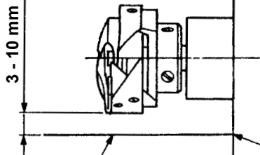
Carta per verificare gli spruzzi di olio
