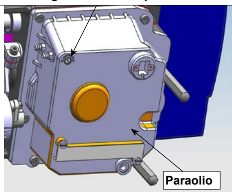
Vite di regolazione della quantità di olio
