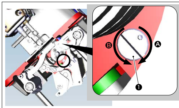
Vite di regolazione della quantità di olio
