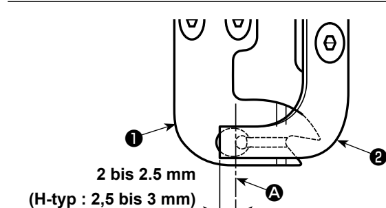
Eingriffszustand des Messers
