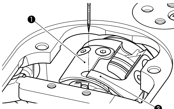
Ausrichtungszustand des vorspringenden Teils des Schleifenspreizmessers und Fadenmessers
