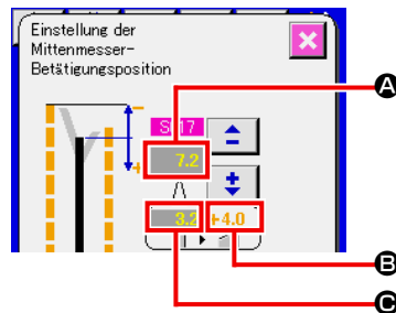
Einstellbildschirm für Mittenmesser-Betätigungsposition (Bildschirm B)
