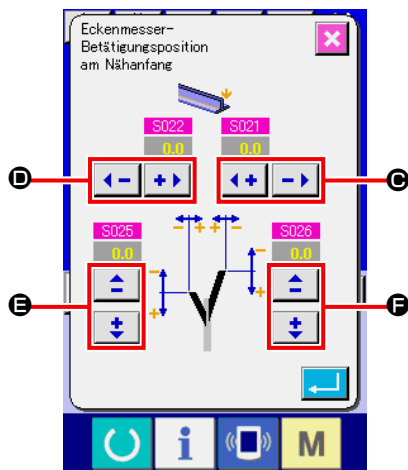
Einstellbildschirm für die Eckenmesser-Betätigungsposition am Nähfang (Bildschirm A)
