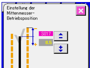
Einstellbildschirm für Mittenmesser-Betätigungsposition (Bildschirm A)
