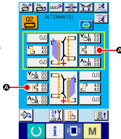
Wechselnähtmodus
