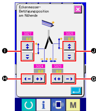
Einstellbildschirm für die Eckenmesser-Betätigungsposition am Nähende (Bildschirm B)
