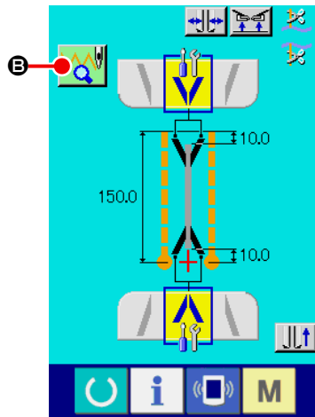
Eckenmessereinstellungs-Nähbildschirm (A)
