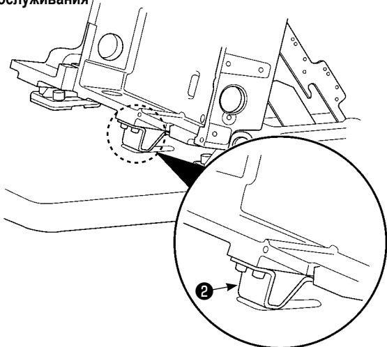
Положение швейной машины для технического обслуживания
