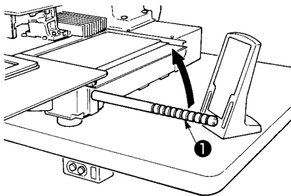
Posizione di manutenzione della macchina per cucire
