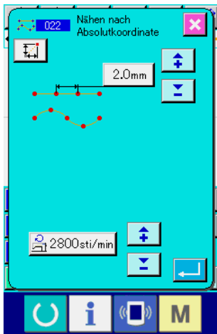
Nähposten-Einstellungsbildschirm
