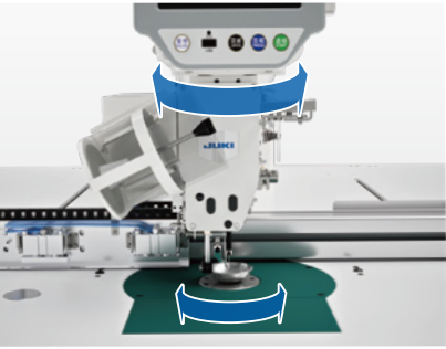
頭部と釜部は同期回転
