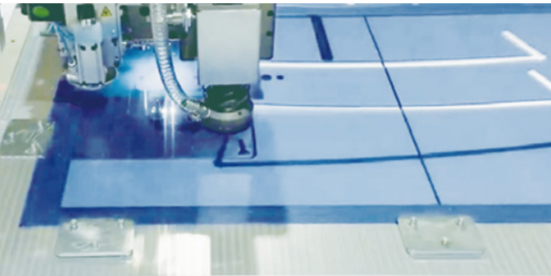
ミーリング時加工工程
