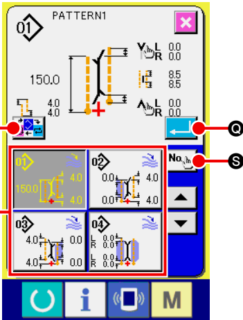
Doğrudan erişimli dikiş çeşidi seçme ekran görünümü (B ekranı)
