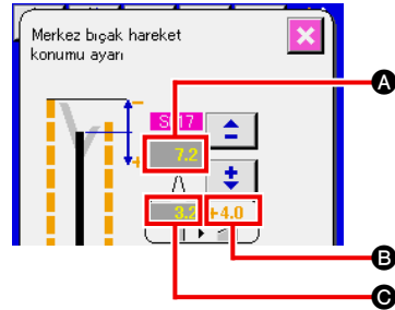
Orta bıçak hareket konumu ayarı ekran görünümü (B ekranı)
