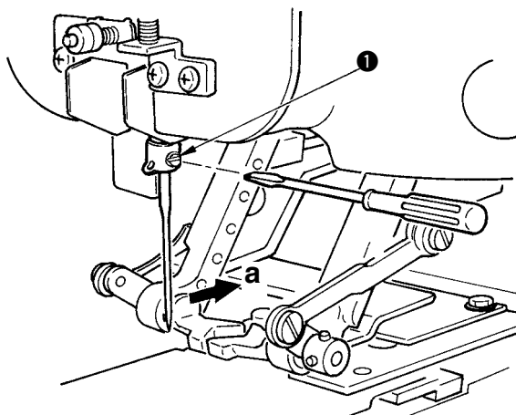
[Nadelinstallationszeichnung]
