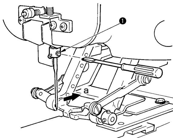
[ 机针安装图 ]
